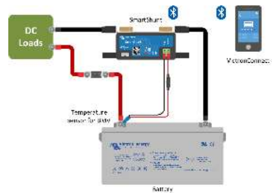
Mäta batteritemperatur
